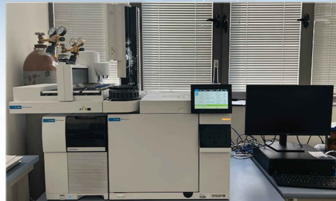
Двудименсионален (2D) газов хроматограф с мас-спектрометричен и пламъчно-йонизационен детектори (2D-GC-FID-MS)
